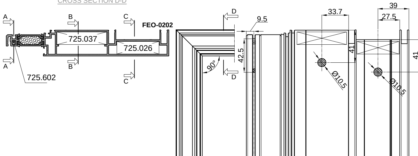
PRESJEK D-D CROSS SECTION D-D
