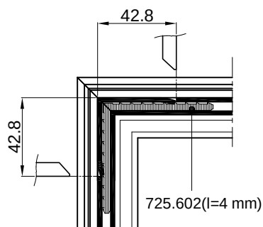
PRESJEK A-A CROSS SECTION A-A
