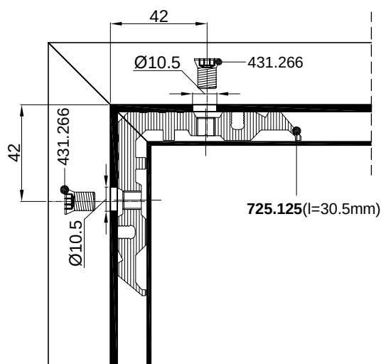
PRESJEK C-C CROSS SECTION C-C
