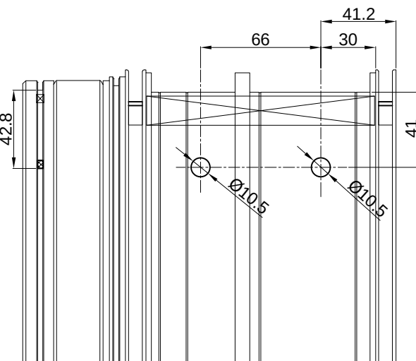
PRESJEK B-B CROSS SECTION B-B
