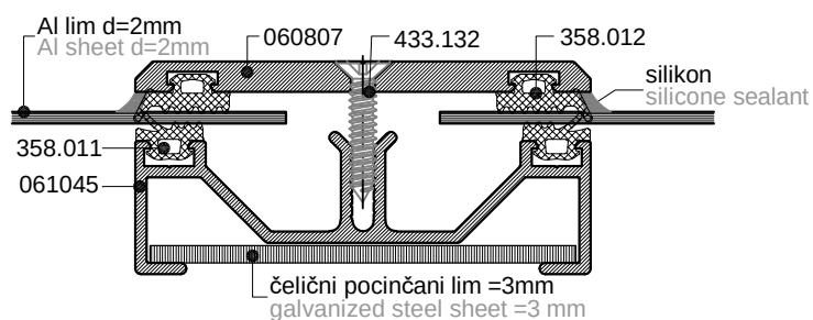
Presjek A-A M 1:2 Cross section A-A M 1:2
