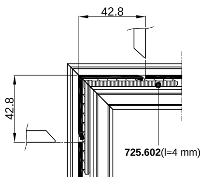
PRESJEK A-A CROSS SECTION A-A
