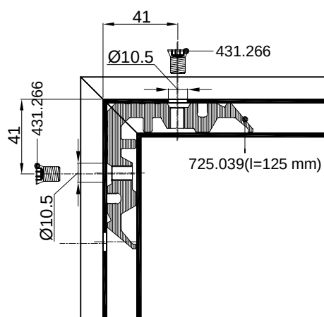
PRESJEK B-B CROSS SECTION B-B
