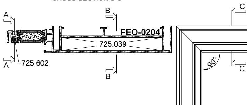
PRESJEK C-C CROSS SECTION C-C
