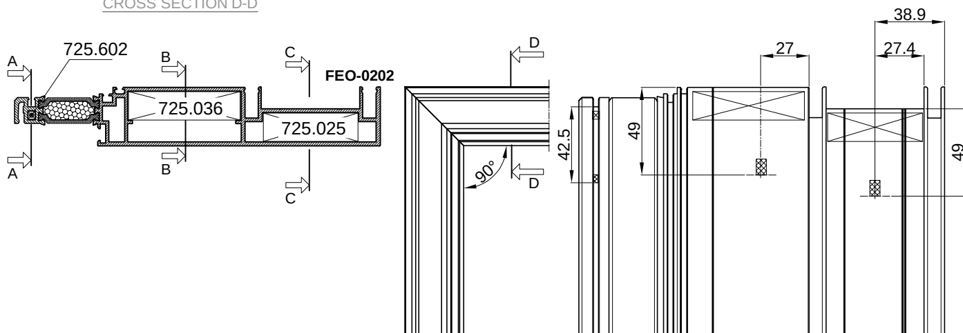
PRESJEK D-D CROSS SECTION D-D
