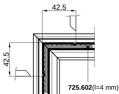
PRESJEK A-A CROSS SECTION A-A
