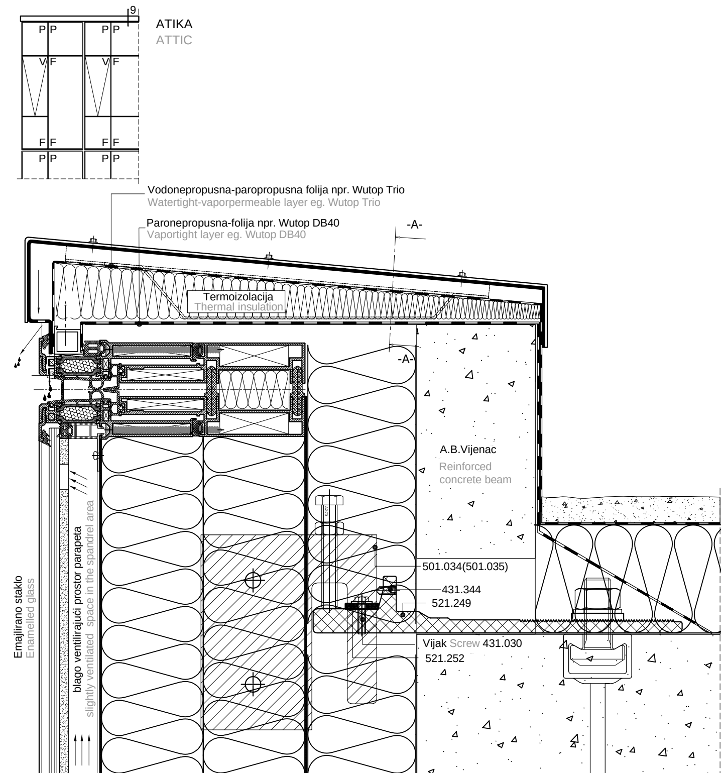
Presjek A-A M 1:2 Cross section A-A M 1:2
