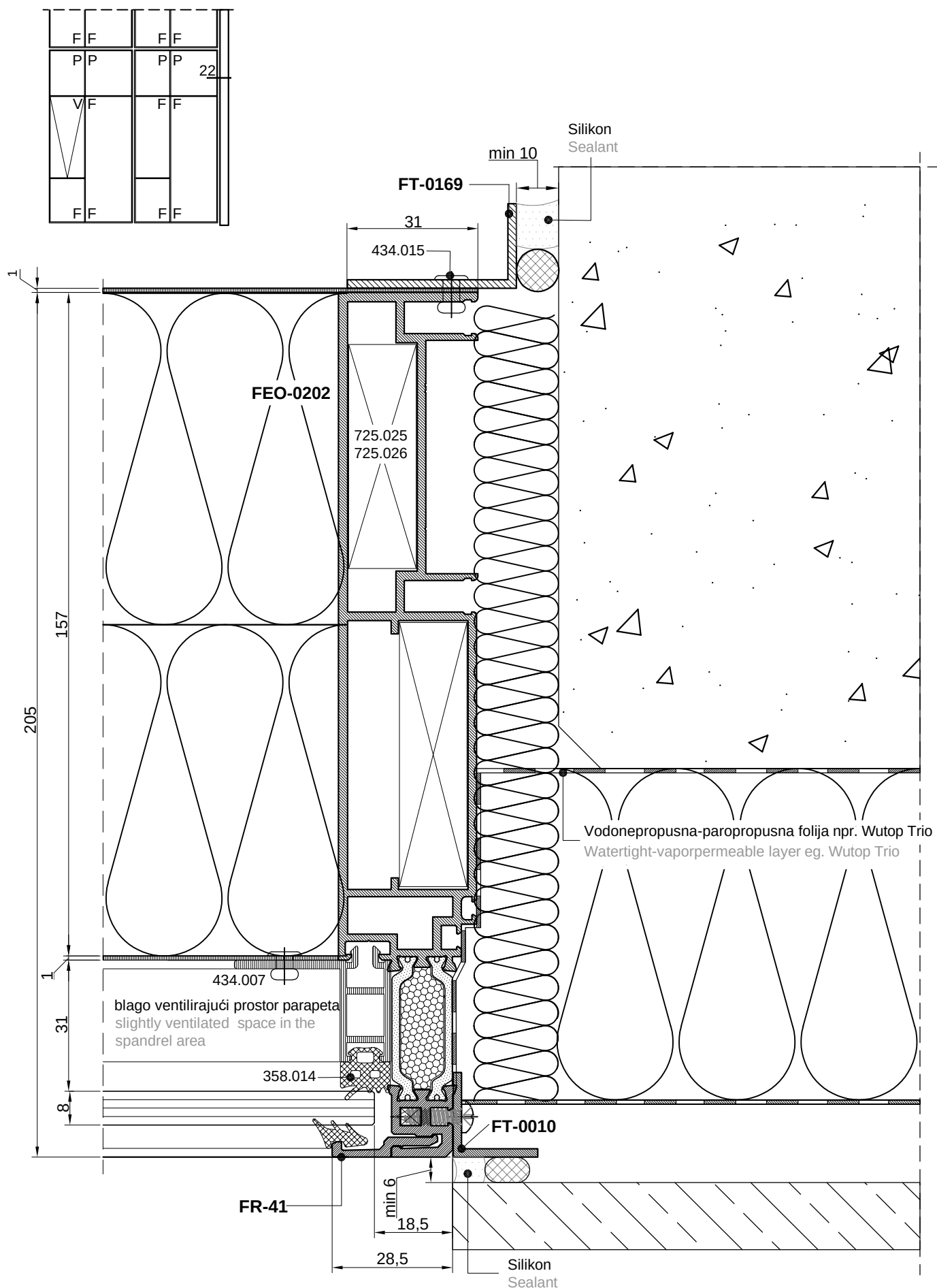
Spoj sa zidom - Presjek 22-22 Wall connection Cross section 22-22
